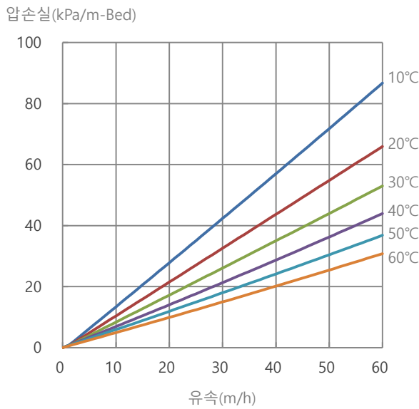
그림 3. TRILITE® UPRA100U Cl-형 압손실
