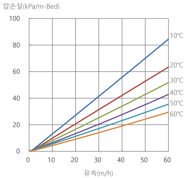
그림 4. TRILITE® UPRA100U OH-형 압손실
