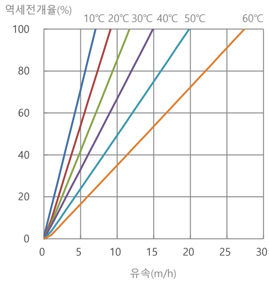
그림 2. TRILITE® UPRA100U OH-형 역세전개
