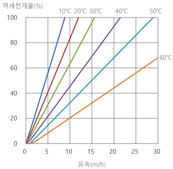
그림 1. TRILITE® UPRA100U Cl-형 역세전개율
