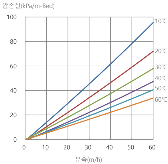
그림 3. TRILITE® MC-08 Na + 형 압손실
