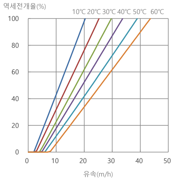
그림 2. TRILITE® MC-08 H + 형 역세전개율
