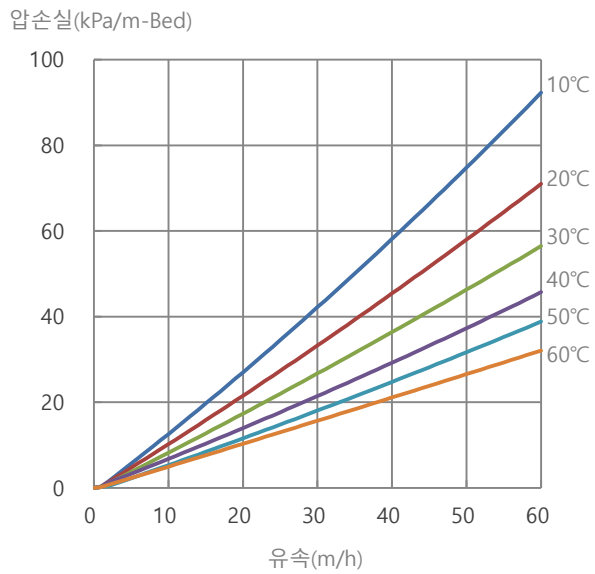
그림 4. TRILITE® MC-08 H + 형 압손실
