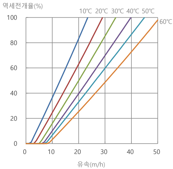
그림 1. TRILITE® MC-08 Na + 형 역세전개율
